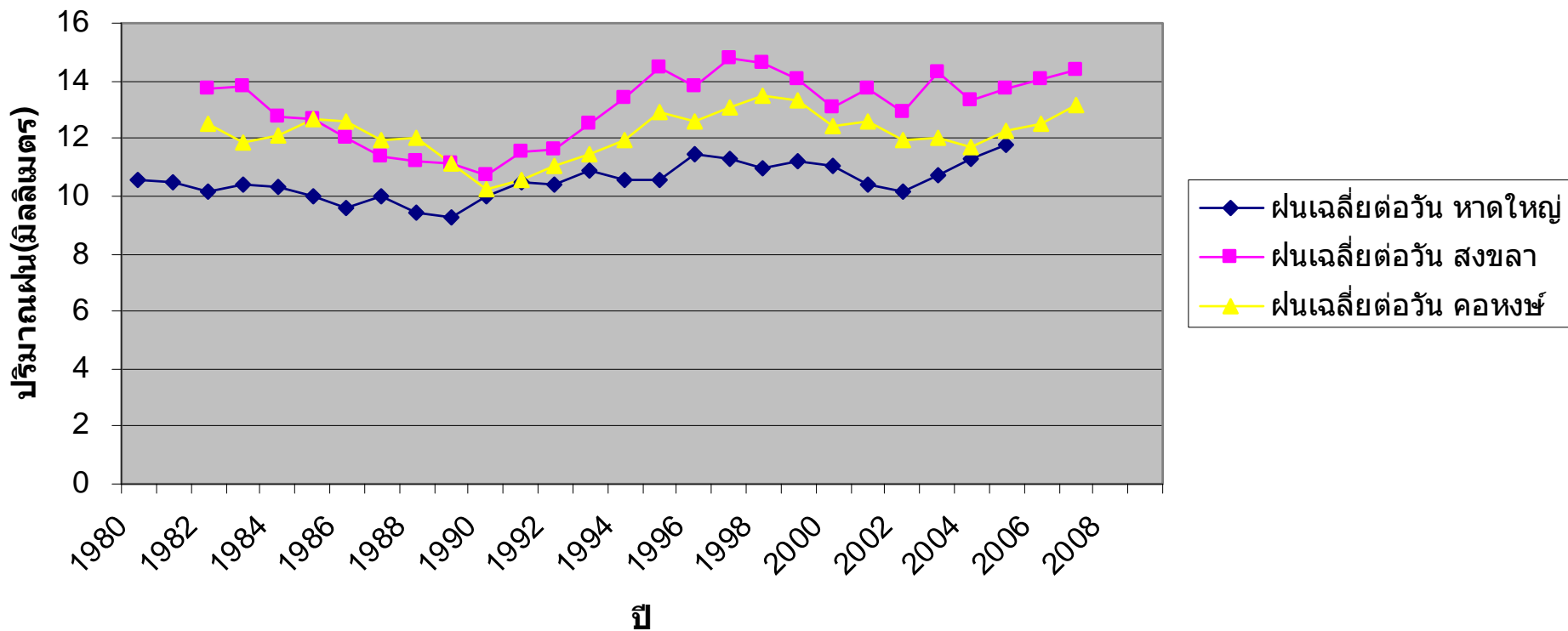
กราฟแสดงปริมาณฝนเทียบกับจำนวนวันที่ฝนตกเฉลี่ย 5 ปี
