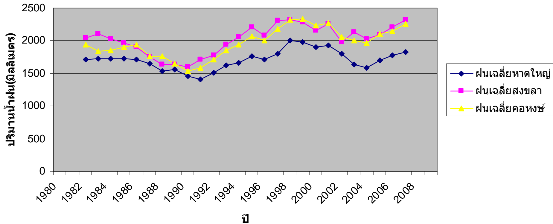
กราฟแสดงปริมาณฝนเฉลี่ย 5 ปี
